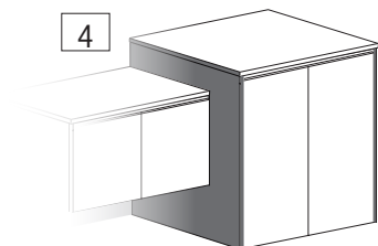
2 fianchi di chiusura. 2 Jous terminales. 2 closing sides. 2 Seitenteile.
